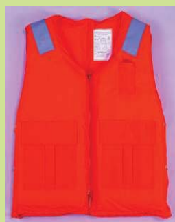
型號：YD-9021 品名：救生衣 浮力：7.5 公斤 EPE 泡沫塑膠
