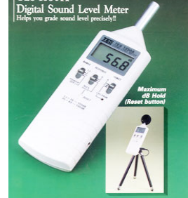
型號：TES-1350A 品名：噪音計 A、C 權衡網 範圍：35-130dB
