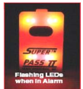
型號：Super Pass II 品名：生命警報器 本質安全防爆，行動感 測、溫度感測、重量輕 18-23 秒人員無動作發 出警報 NFPA1982，UL913 Class1 GroupsA,B,C,D
