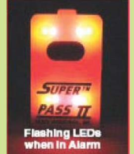
型號：Super Pass II 品名：生命警報器 本質安全防爆，行動感測、 溫度感測、重量輕 18-23 秒人員無動作發出警報 NFPA1982，UL913 Class I Groups A,B,C,D
