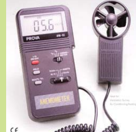
型號：AVM-03 品名：風速風溫計 範圍：風速 0.3-45 M/S 範圍：風溫 0-60°C
